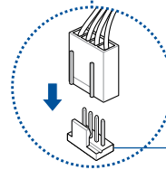
Motherboard fan header
